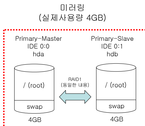
[그림 B1-2] 이번 실습에서 구성할 RAID1
