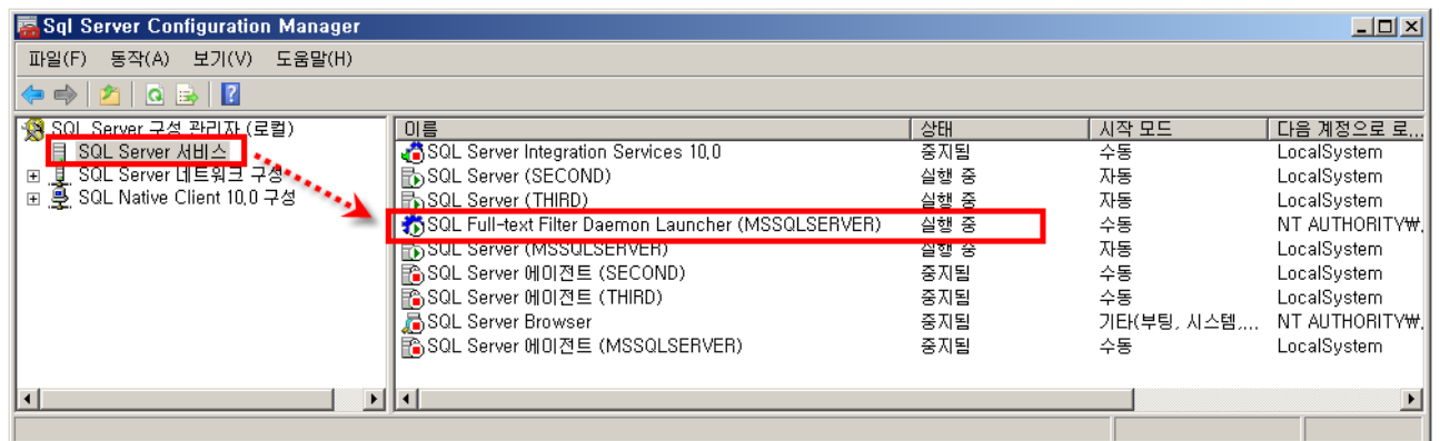
[그림 2-3] SQL Full-text Filter Daemon Launcher가 실행 중인 상태 $$ 02-n03.bmp $$
