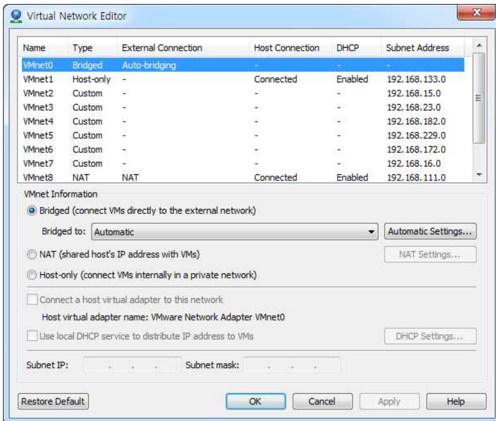
[그림 D-4] VMware Player 3.x에서 Virtual Network Editor 실행
